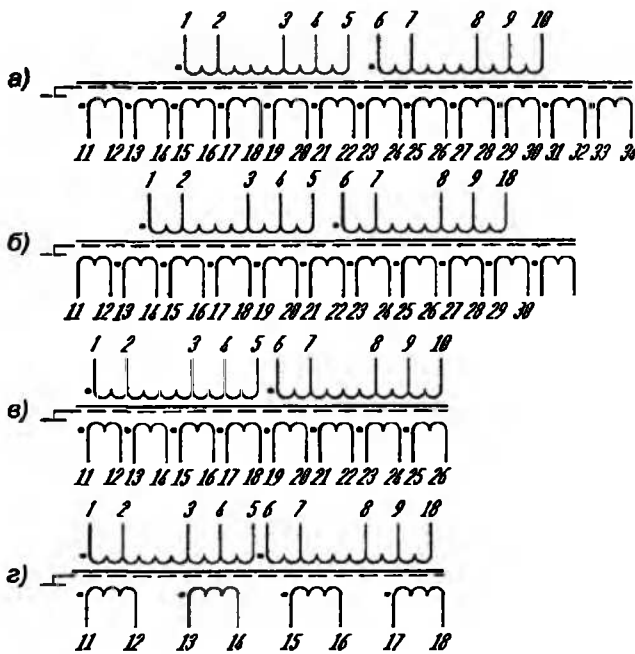
Рис. 2.9. Электрические схемы трансформаторов типа ТПП2 с частотой питающей сети 50 Гц: а) — ТПП2; б) — ТПП2 2; в) — ТПП2 3; г) — ТПП2 5
