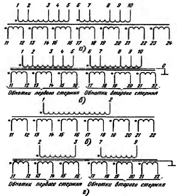
Рис. 2.10. Электрические схемы трансформаторов типа ТПП с частотой питающей сети 50 Гц: а) — броневой конструкции с напряжением 127/220 В; б) — стержневой конструкции с напряжением 127/220 В; в) — броневой конструкции с напряжением 220 В; г) — стержневой конструкции с напряжением 220 В
