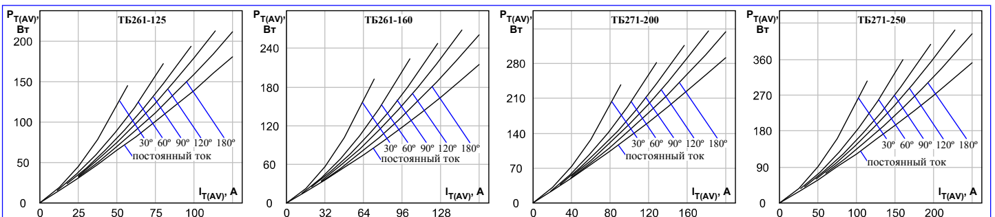
Рисунок 7: Зависимость средней рассеиваемой мощности P_{T(AV)} от среднего тока I_{T(AV)} прямоугольной формы частотой 50 Гц при различных углах проводимости и постоянного тока.
