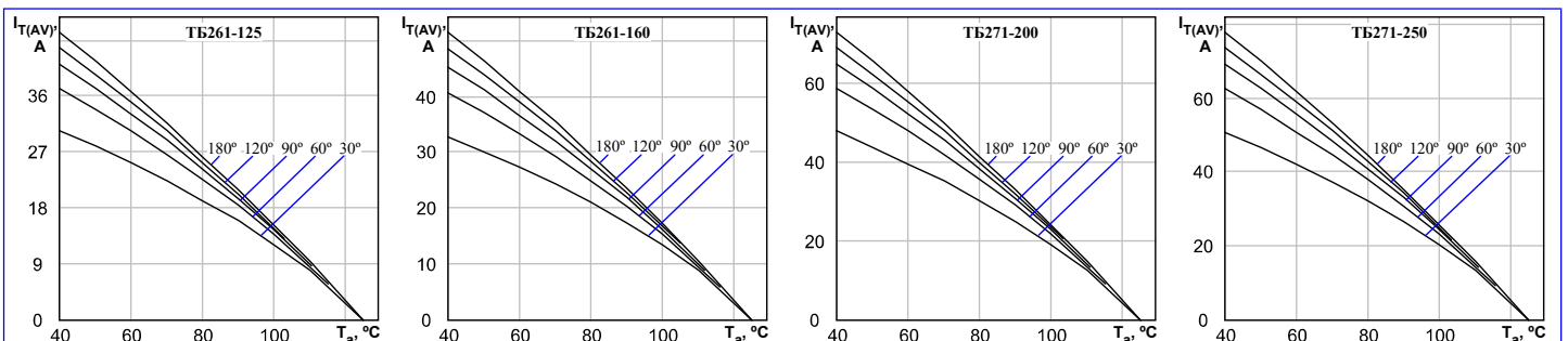
Рисунок 8: Зависимость допустимого среднего тока I_{T(AV)} синусоидальной формы частотой 50 Гц при различных углах проводимости от температуры окружающей среды T_a при естественном охлаждении TB271 на OP281-110 и TB261 на OP171-80.
