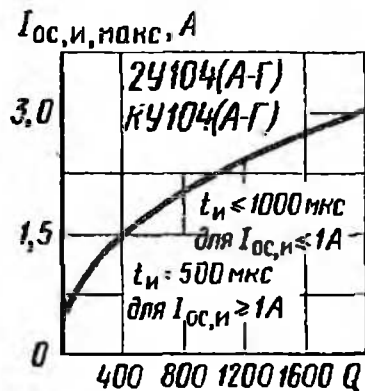
Зависимость допустимого импульсного тока в открытом состоянии от скважности
