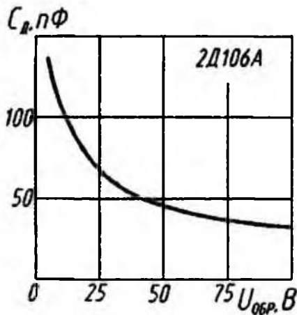
Зависимость общей емкости диода от напряжения
