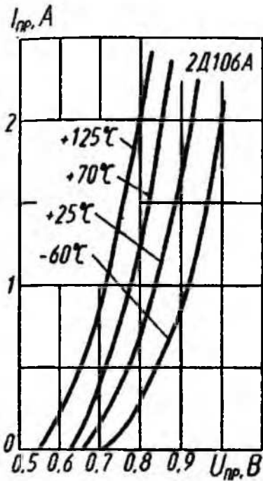
Зависимости прямого тока от напряжения
