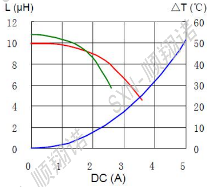
SMRH8D58-100N
