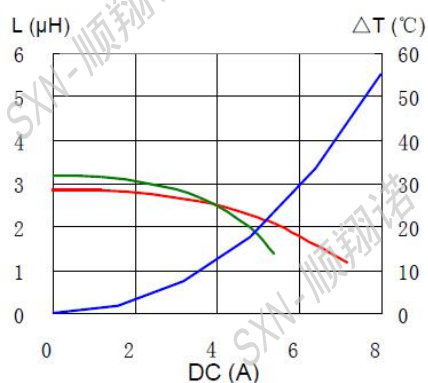
SMRH8D58-2R8N
