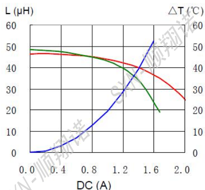
SMRH8D38-150N
