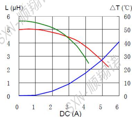
SMRH8D58-5R0N
